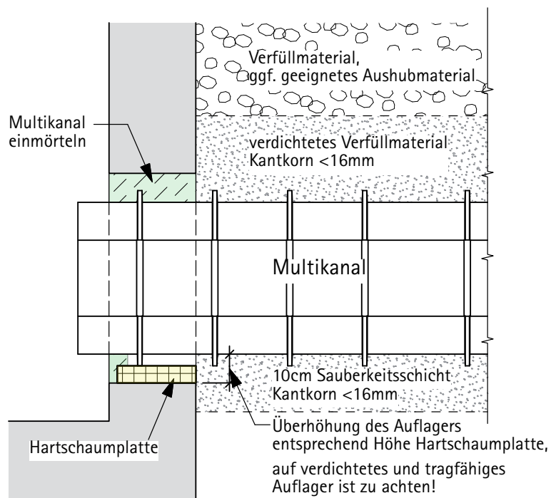
Vertikalschnitt Einführung Multikanal in Kabelschacht
